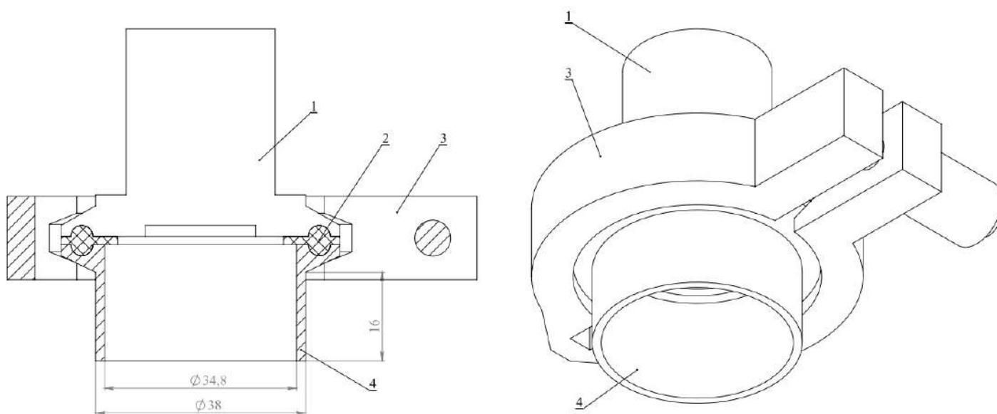
Рисунок Г.5 — Рекомендуемые монтажные гнезда для преобразователей с кодами соединительной части 1, 8, A
